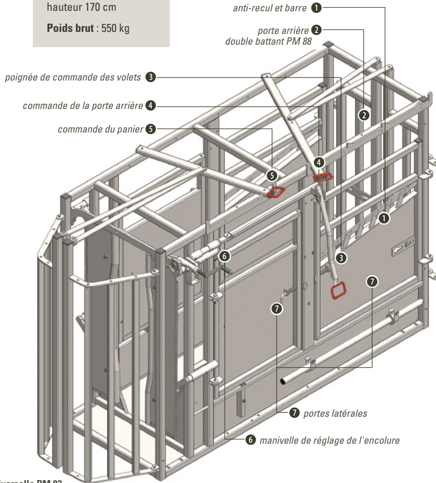
porte universelle PM 83
