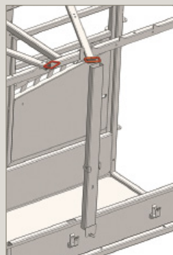
POTEAU CENTRAL démontable pour cage PM 2400
