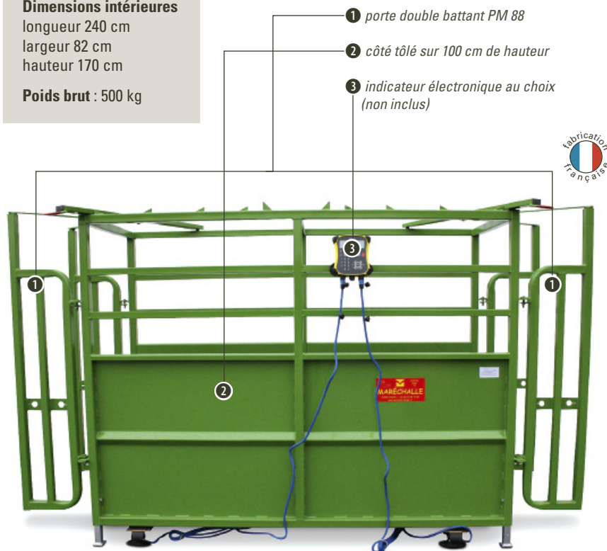
cage pour chevaux
