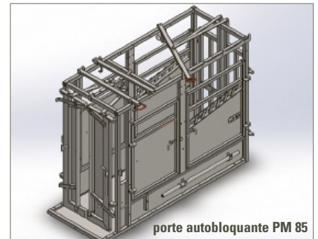
porte cornadis PM 80
