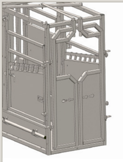
PORTE ARRIÈRE Porte d'insémination PM 82
