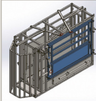
PORTE ARRIÈRE Porte sectionnelle PM 87
