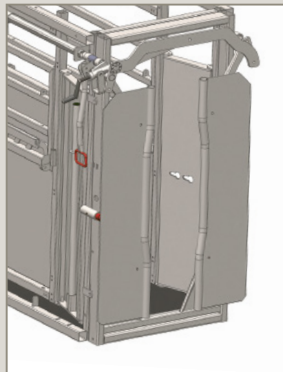
PORTE ARRIÈRE Porte sectionnelle PM 87
